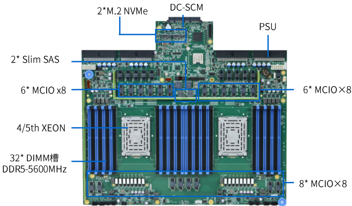
主板
