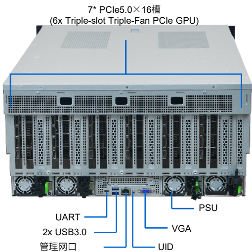
后视图
