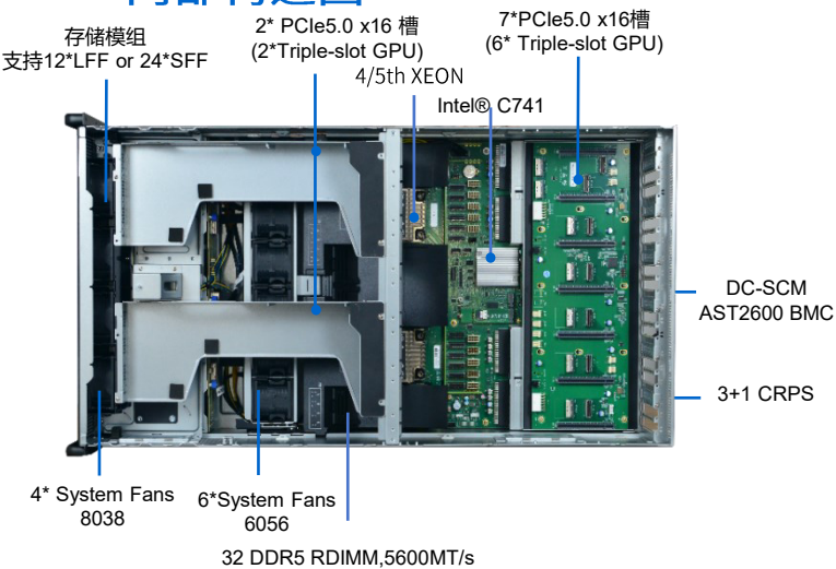
内部构造图
