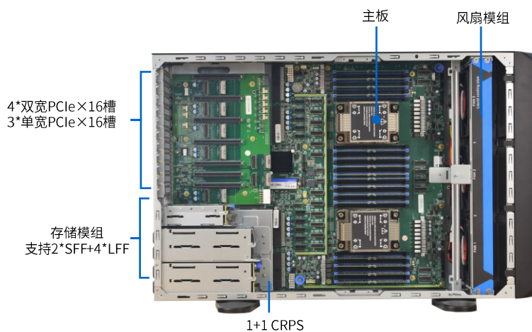
内部构造图
