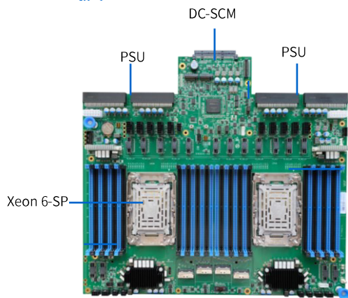
主板
