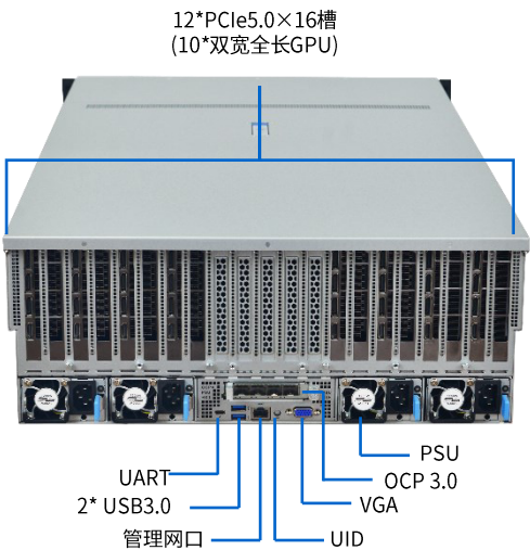
后视图
