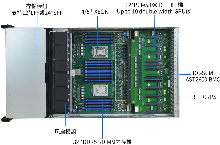
内部构造图
