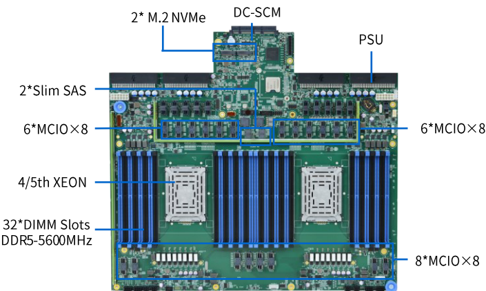
主板
