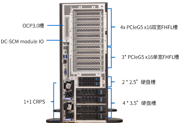
后视图
