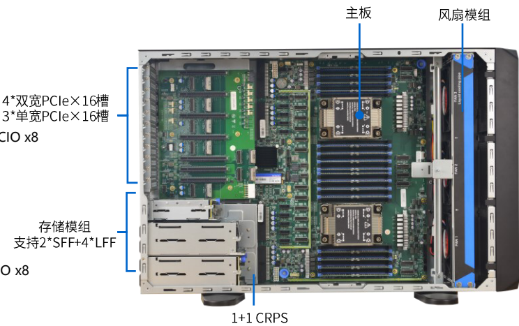
内部构造图
