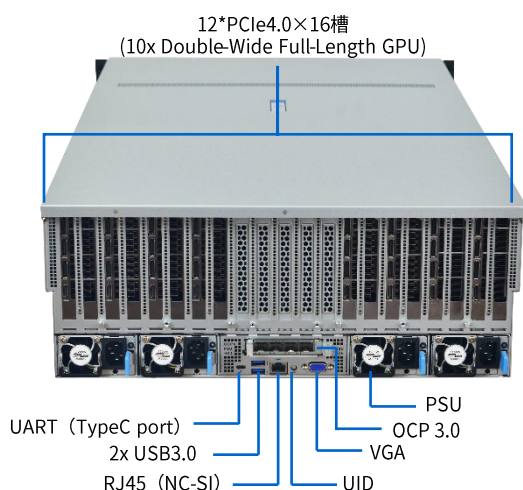
后视图
