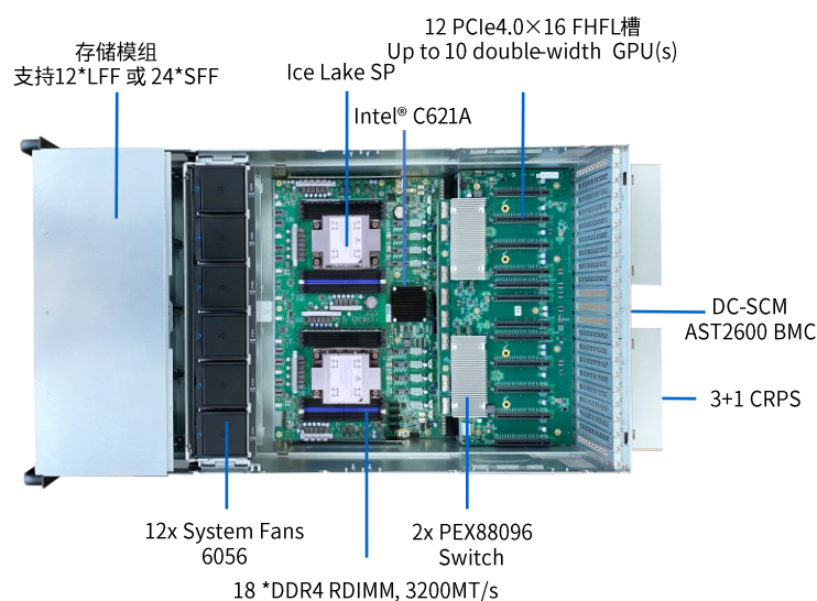
内部构造图
